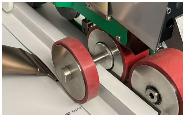
Obr. 8: Detail provedení spoje automatickým svařovacím přístrojem
