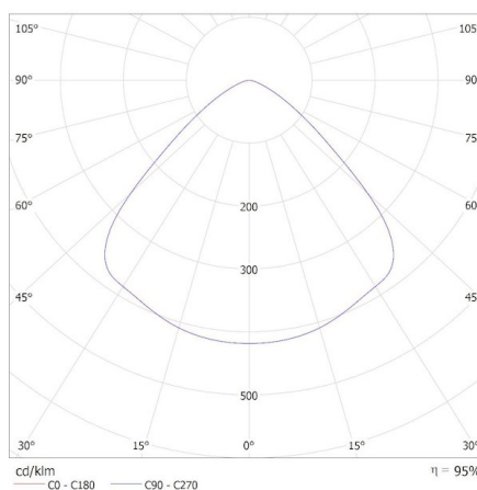
KANLUX S.A. (kat 27163 + 38135) HB PRO STRONG 100W-NW + GRID / Krzywa rozsyłu światła (biegunowo)
