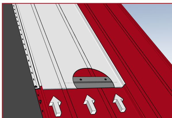
Zavlečení navazujícího šáru krytiny
