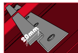
Podtěsnění pomocí lišty
