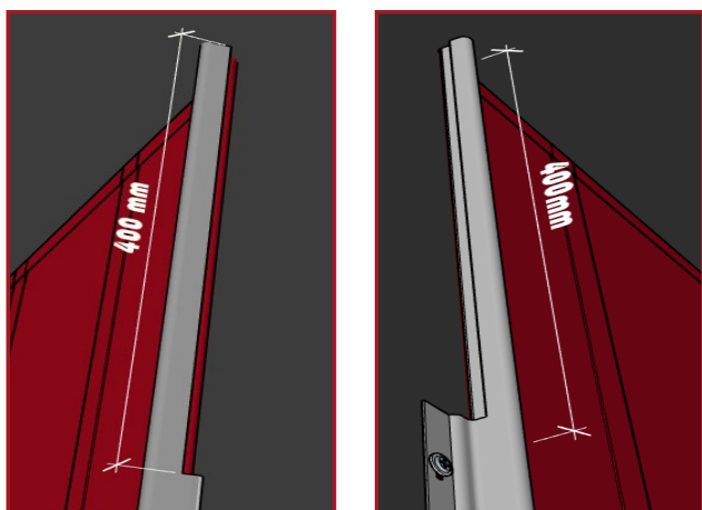
Příprava zámků krytiny pro napojení
