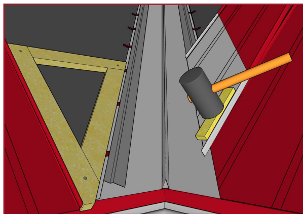
Detail úžlabí
