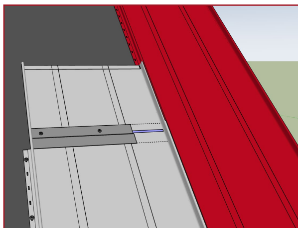
Osazení lišty pro napojení – těsněno EPDM páskou 3x9 mm, nebo tmelem
