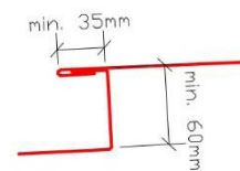
Spádový stupeň 4–10°
