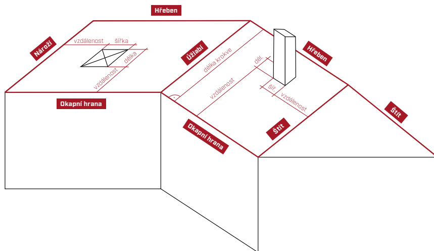
Obrázek 3: Schéma rozměření střechy pro vyhotovení kladečského plánu
