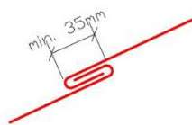
Jednoduchá ležatá drážka ≥ 30°
