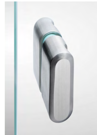
NAVE rozteč 48,5 mm, délka 73 mm Z8023006
